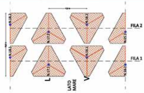
Piano di posa: Tabella georeferenziata di posa dei moduli
